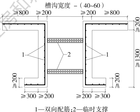
图 4.1.1-2 “[”形导墙示意图(单位:mm)
