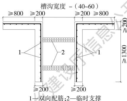
图 4.1.1-1 倒“L”形导墙示意图(单位:mm)
