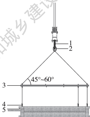
1—起重机械吊钩;2—吊环;3—框式吊梁; 4—吊具;5—吊点承力件
