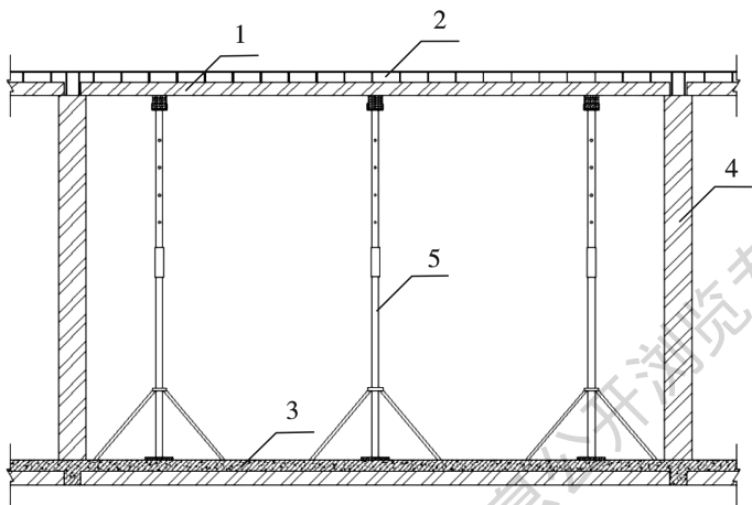
1—叠合楼板预制底板;2—叠合楼板现浇层;3—下部叠合楼板; 4—施工完毕的墙或柱;5—可调独立支撑
