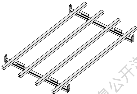
图 4.4.4 构件水平叠放托架示意
