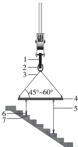
1—起重机械吊钩;2—吊环;3—起重吊索; 4—框式吊梁;6—吊具;7—吊点承力件
